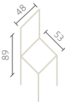
9230 Kitchen wood Impilabile
