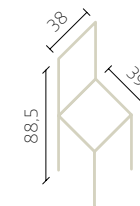
9020 Chiavarina rinforzata PP Impilabile
